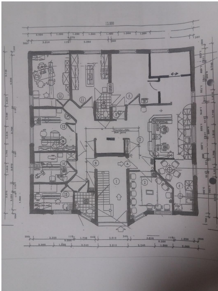
Abbildung 7: Grundriss
